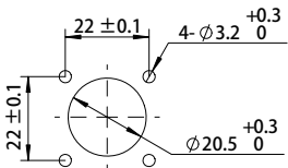
四孔座子安装孔尺寸
