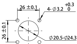
四孔座子安装孔尺寸
